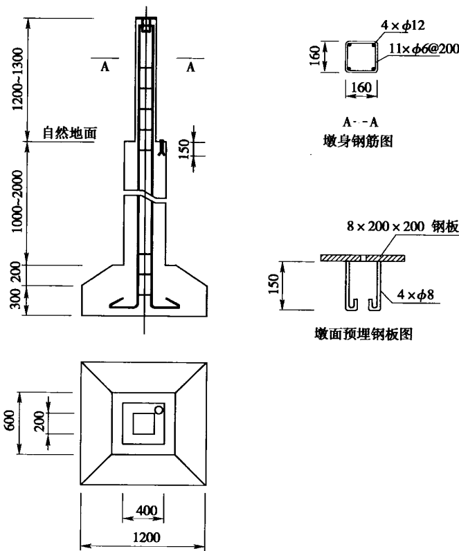
图 B. 3. 1 变形监测观测墩图(mm)
